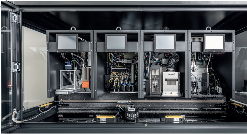
Module der NextFactory-Anlage basierend auf einer Kombination von 3D-Druck und Mikromontage.
